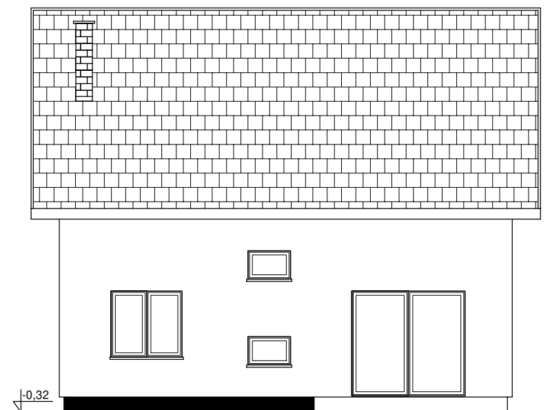
ELEWACJA TYLNA PÓŁNOCNO-ZACHODNIA
