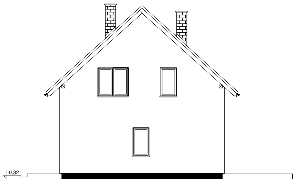
ELEWACJA PÓŁNOCNO-WSCHODNIA
